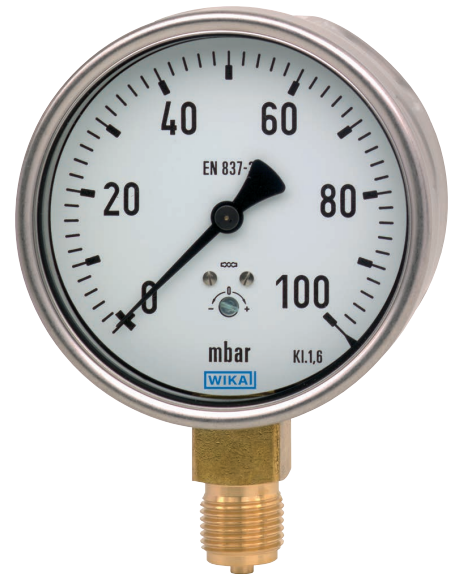
Manómetro con muelle de membrana elástica modelo 612.20
