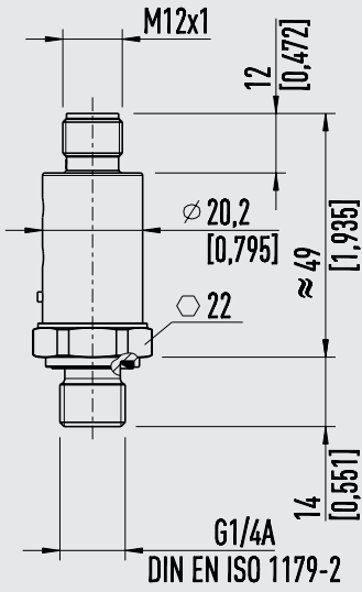
Con conector circular M12 x 1
